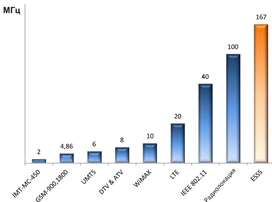
РИСУНОК 14 Спектр, занятый радиосистемой (БС), для определенных радиотехнологий, режимов связи и типов систем, МГц
