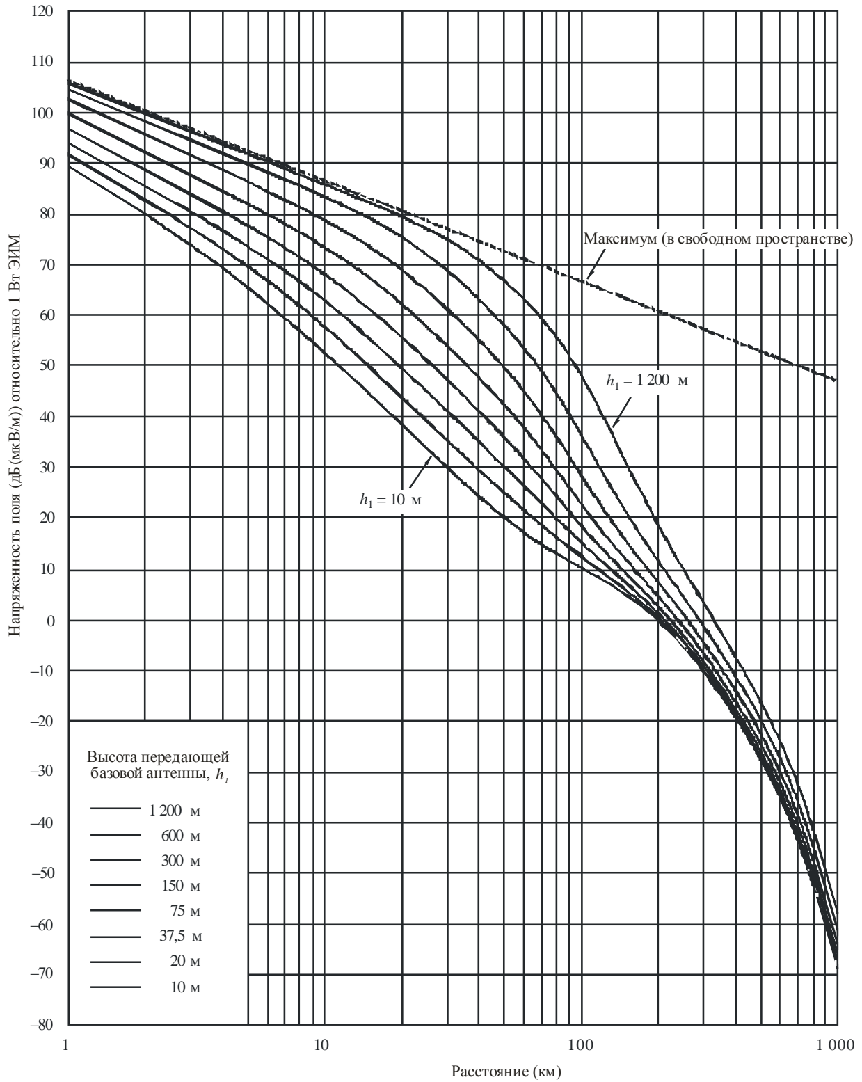
Кривые распространения в диапазоне частот 30–300 МГц
