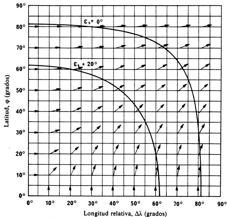
FIGURA 3 — Variación del ángulo de polarización recibido en la Tierra
