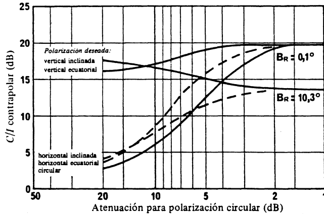
FIGURA 1 – Disponibilidad de relación C/I contrapolar en el borde de la zona de cobertura, entre satélites coubicados que dan servicio a zonas de haces adyacentes (Se supone que las antenas están perfectamente alineadas)
