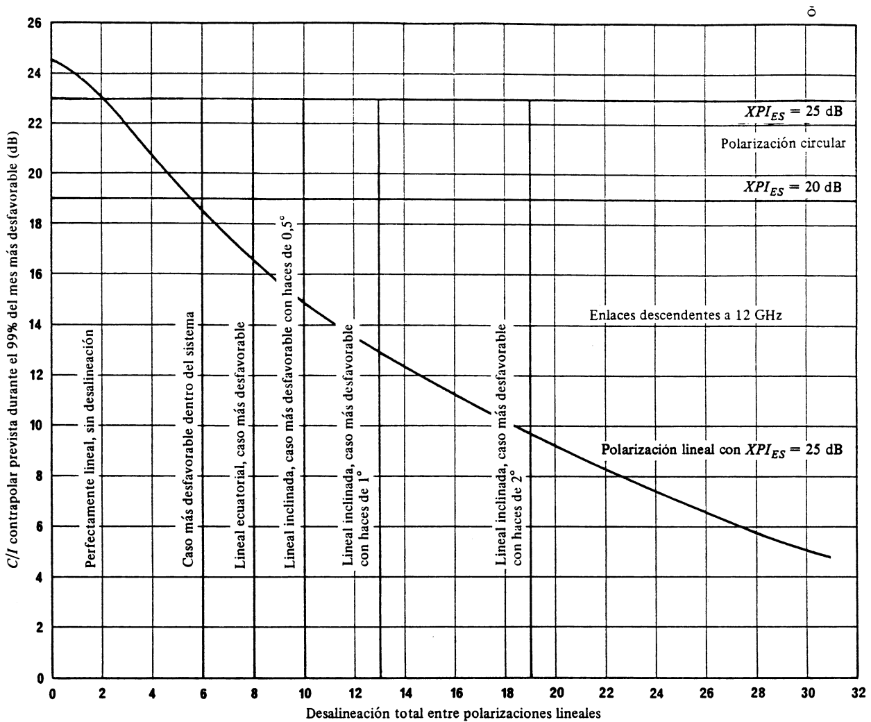
FIGURA 2 – C/I contrapolar en condiciones de cielo despejado entre haces de satélites adyacentes transmitidos desde un satélite a una estación terrena situada en el punto común de los contornos a -3 dB (Se ilustran el caso más favorable de polarización lineal ecuatorial y de polarización circular y el caso más desfavorable de polarización lineal inclinada)
